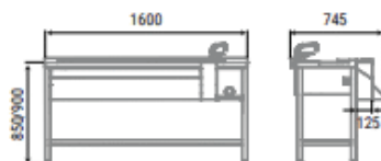
Opcional, 2º carril para botellas, mod. CR-160
